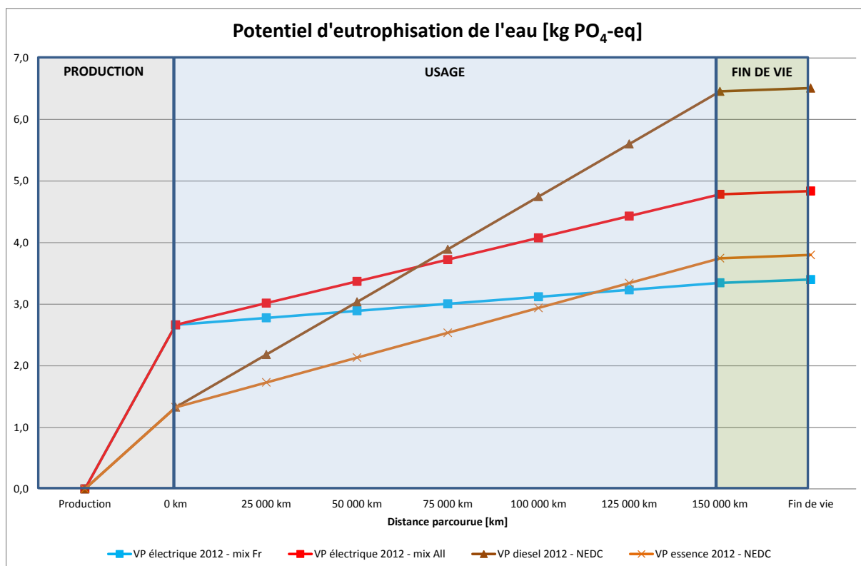
Figure 1-15 : Domaines de pertinence environnementale du véhicule électrique (France et Allemagne) comparés au véhicule thermique pour le potentiel d'eutrophisation en 2012
