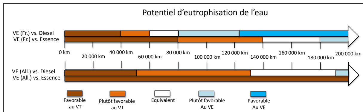
Figure 1-17 : Domaines de pertinence environnementale du véhicule électrique (France et Allemagne) comparés au véhicule thermique pour le potentiel d'eutrophisation de l'eau en 2012
