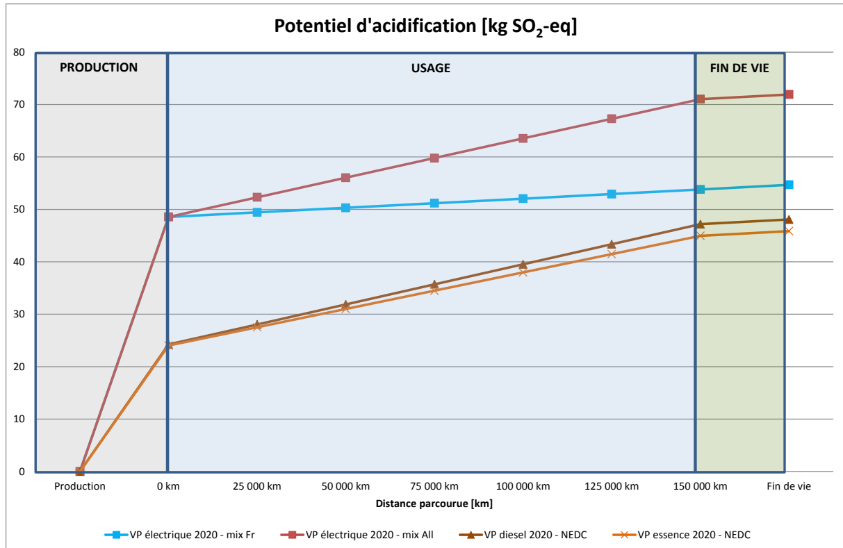
Figure 1-12 : Potentiel d'acidification pour les véhicules électriques français et allemand et les véhicules thermiques essence et diesel à l'horizon 2020 selon le scénario de référence
